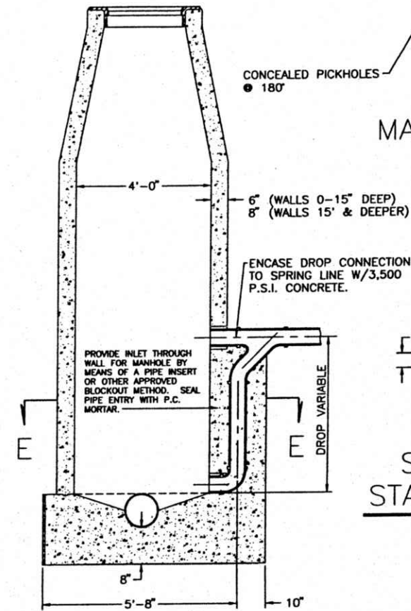
SECTION D-D
